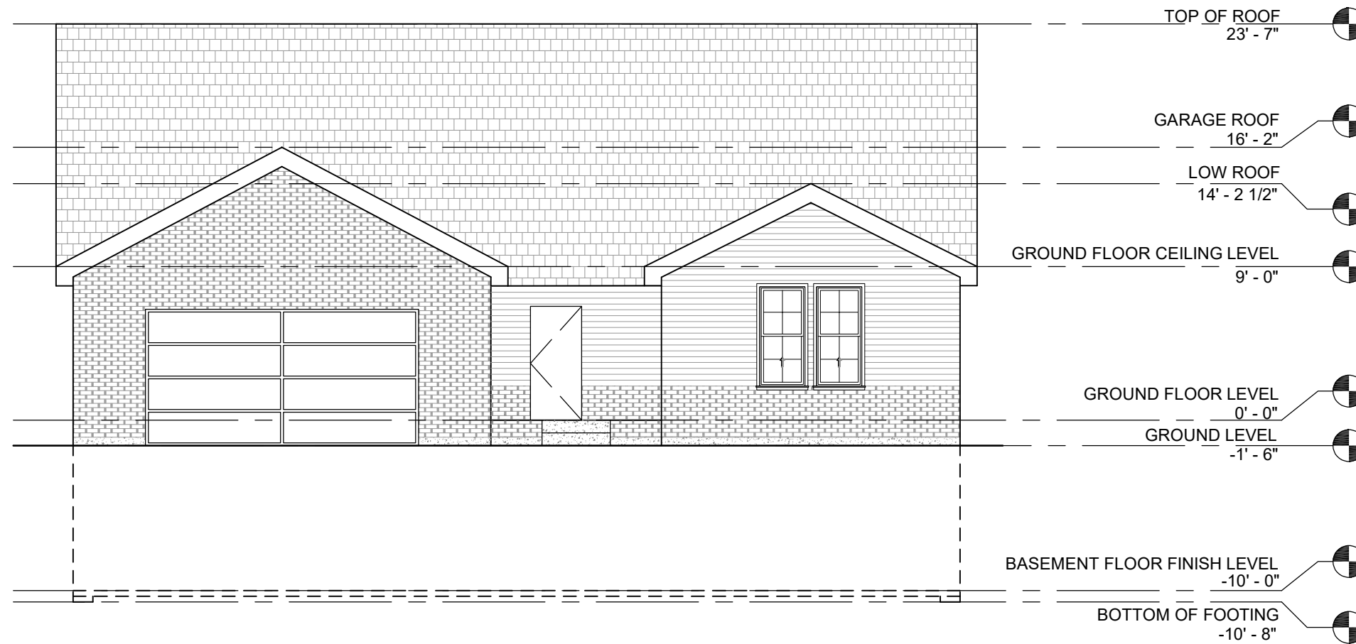
1 FRONT ELEVATION Scale: 1/8"=1'-0"
